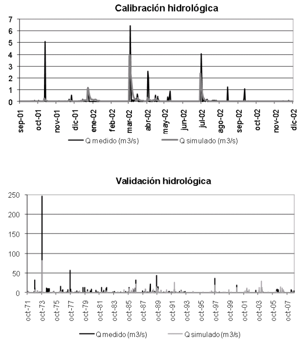
Fig.2. Resultado de la calibración y de la validación hidrológica.
