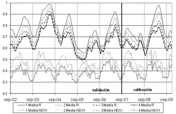
Fig.4. Resultado de calibración y validación del modelo descrito por la Ec. (2). En negro los valores de R, en gris los valores de NDVI medios para cada clase. Las clases son ordenadas desde la menos insolada a la más insolada.
